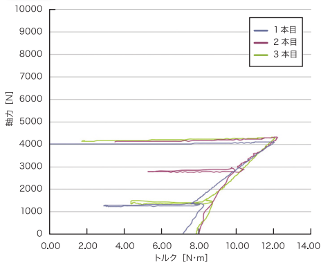
1 タップタイト 2000 三価クロメートめっき (下穴径φ7.30)
