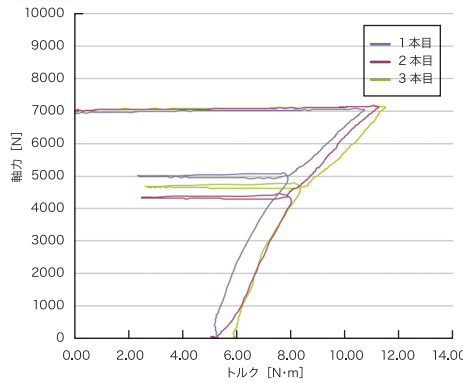
2 タップタイト 2000 三価クロメート+フリックス 009 (下穴径φ7.30)
