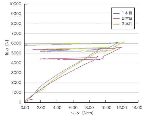
3 小ねじ 三価クロメートめっき (M8 タップ穴)
