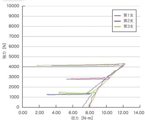
轴力试验结果
