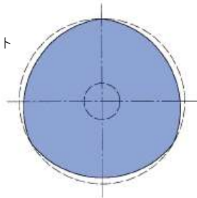
ねじ断面
